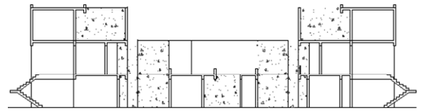
مقطع عرضي في المبنى
