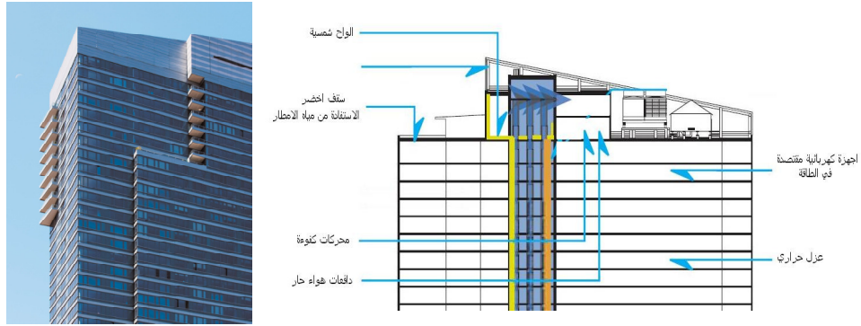
شكل (5): مبنى (Helena) السكني في نيويورك المصدر (Companies, 2008, pp125-127) .
